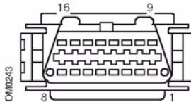
Presa diagnostica J1962
