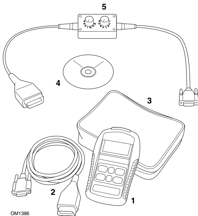
Kit Easycheck di TRW
