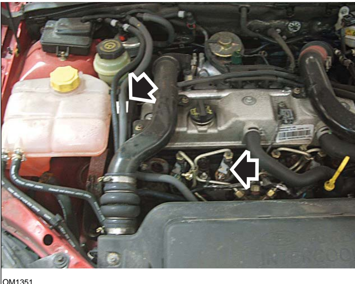
OM1351 Etiqueta de inyectores y cabeza de inyector indicadas con flechas: Vista frontal
