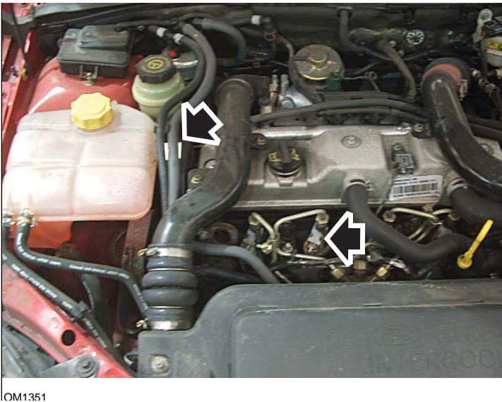
OM1351 Einspritzdüsen-Label und Düsen spitze mit Pfeil gekennzeichnet - Frontansicht
