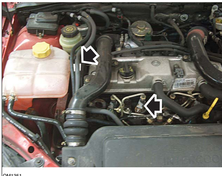
Étiquette et tête d'injecteur indiquée par une flèche sur l'illustration - vue de face
